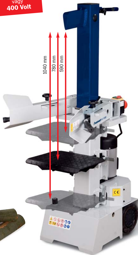
HS 7-1000 (400 V) Rönkhasító
